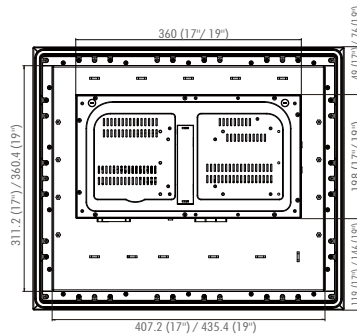
PPC-7917F / 7919F
