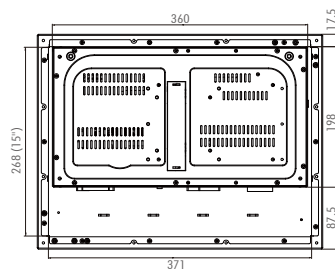
PPC-7915F
